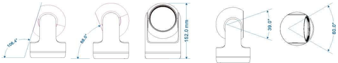
Q90-13P 尺寸图
